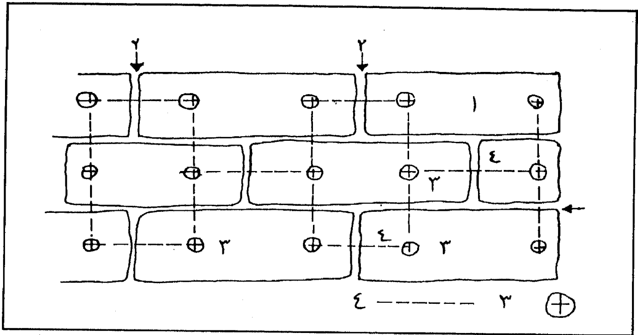
شكل ٢٩ - طريقة رفع الجدران الحجرية هندسيا بواسطة النقط والعلامات.
