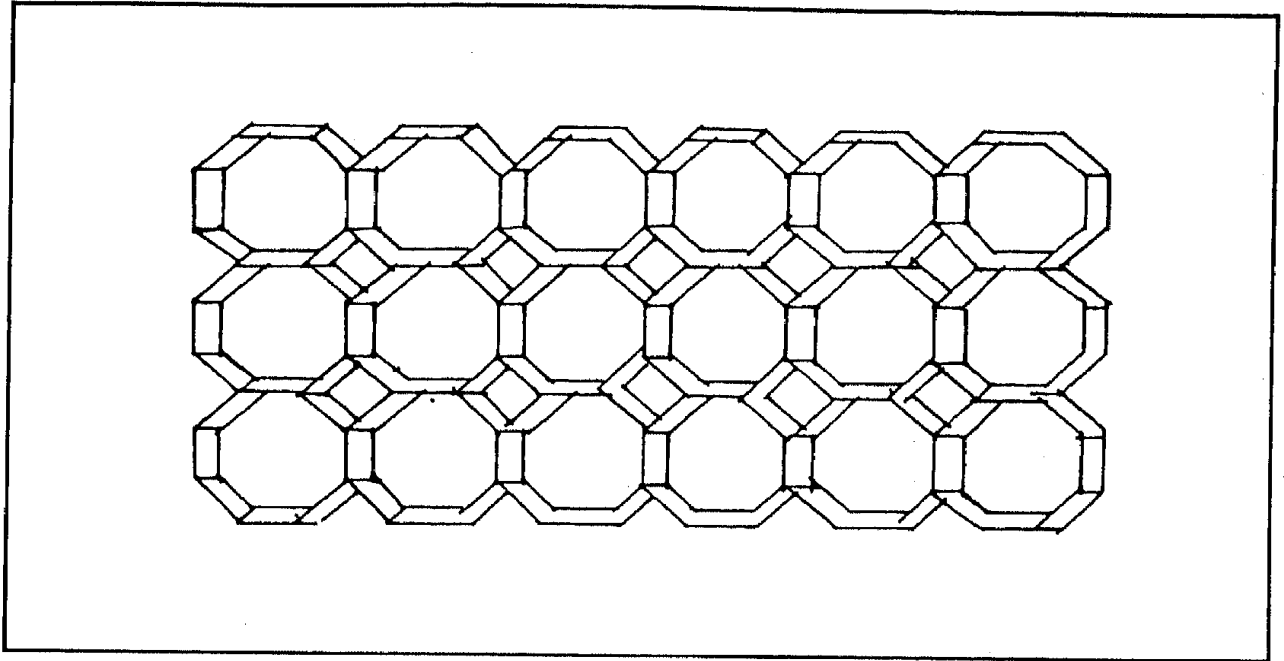
شكل ٤٥ - ورق مقوى على شكل خلية النحل لعزل الرسومات الجدارية.
