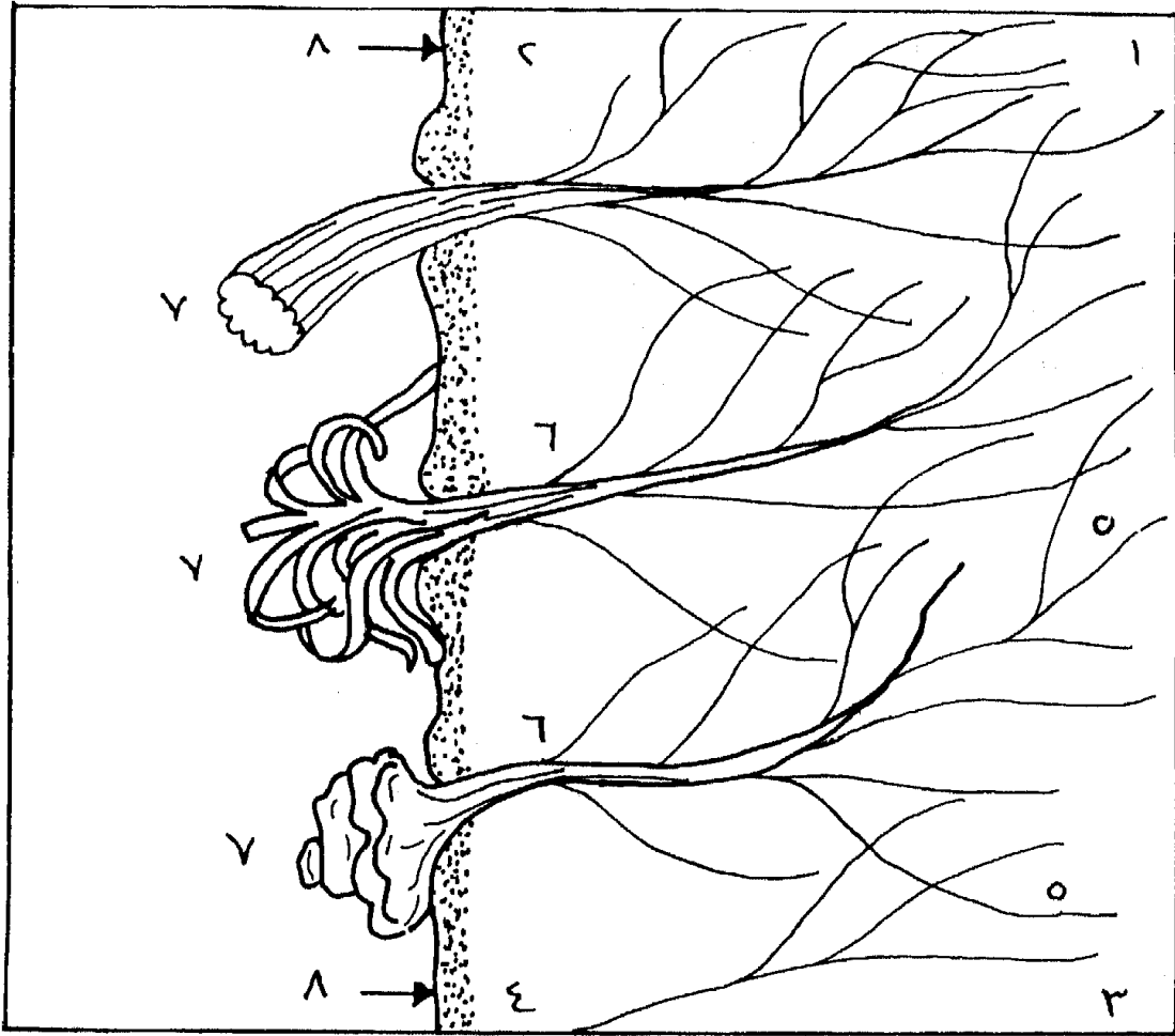
شكل ٣٦ - عملية تزهـر الأملاح في الأحجار.
