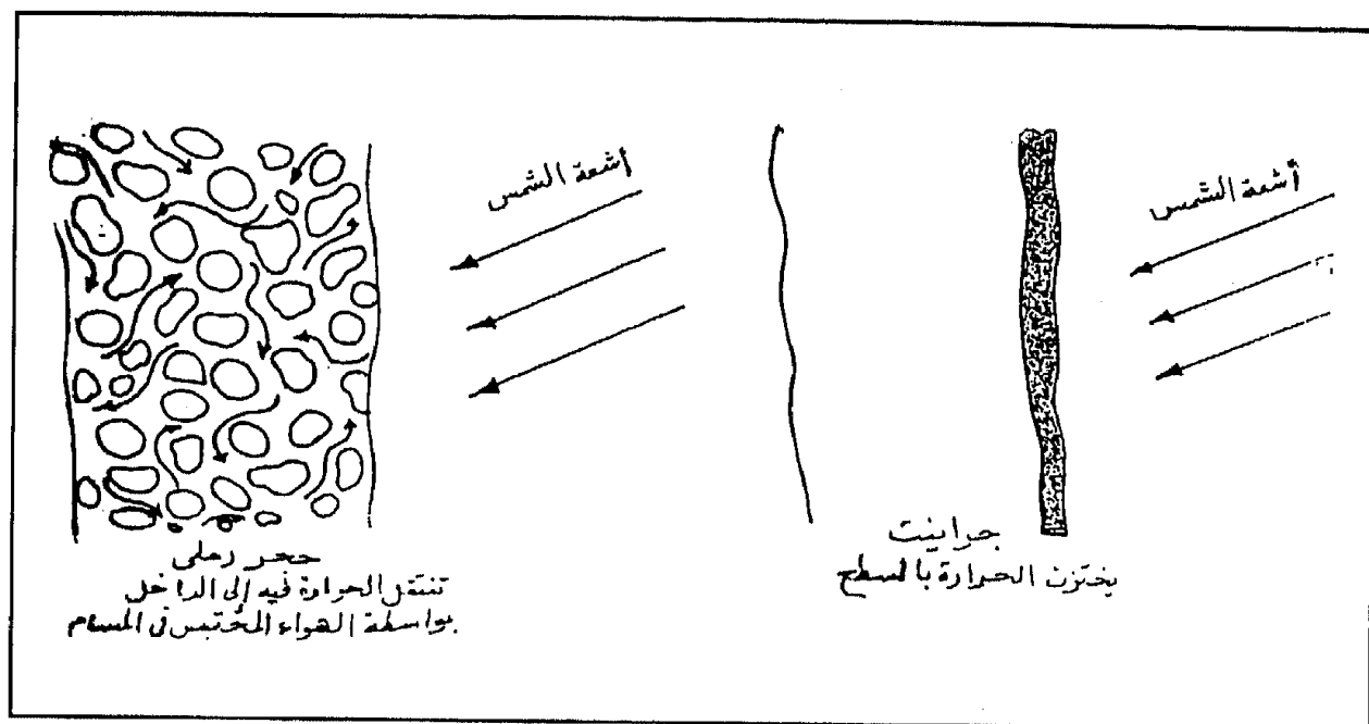
شكل ٣١ - انتقال الحرارة في الأبنية الحجرية.
