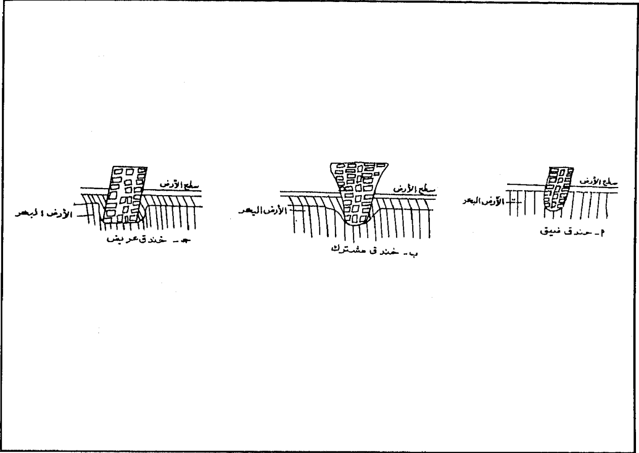
شكل ٢٦ - ثلاثة مقاطعات توضح الأنواع الثلاثة لخنادق الأساسات.
