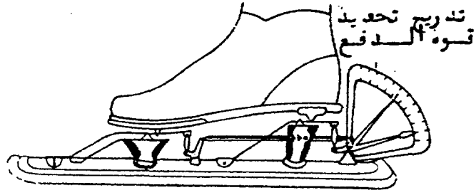
شكل (٧٧) جهاز تسجيل القوى المستخدم في حذاء الانزلاق على الجليد عن (ابلاكوف Abalakov)
