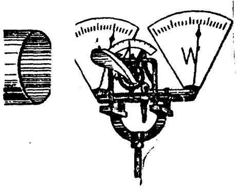
شكل (٦٢) قياس مقاومة تيار الهواء بمقياس صغير
