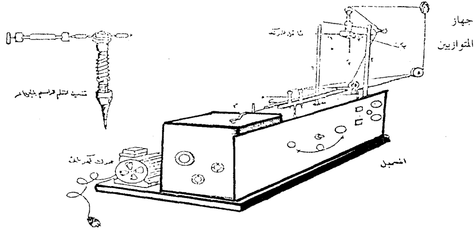
شكل (٨٠) رسم تخطيطى لجهاز تسجيل القوى (عن عادل)
