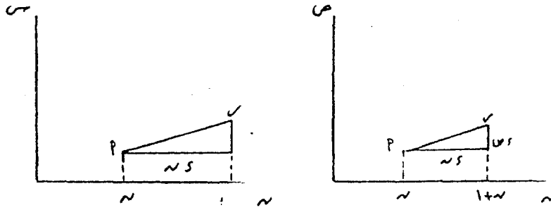
شكل (٢٣) تقسيم الحركة الانتقالية المستوية على مسار منحني إلى مركبتين مستقيمتين أحدهما في الاتجاه (س) والآخر في الاتجاه (ص)
