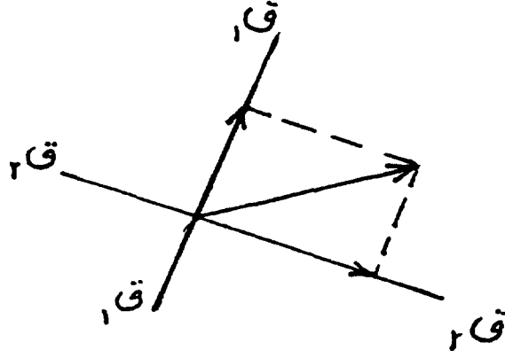
شكل (١٣) متوازي أضلاع القوى
